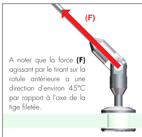
Schéma de la direction de la force agissant sur la rotule
