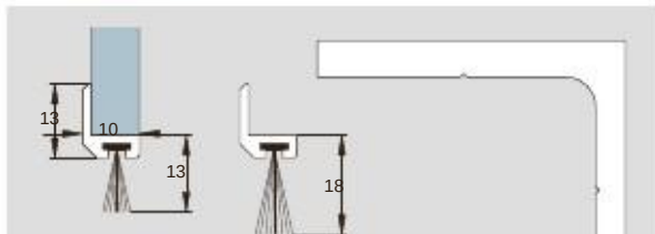
Joint brosse vertical pour espace jusqu'à 13 mm, longueur de stock 3000 mm Réf. 07.400
