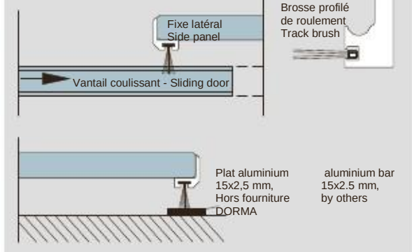
Joint brosse vertical pour espace jusqu'à 18 mm, longueur de stock 3000 mm Réf. 07.402
